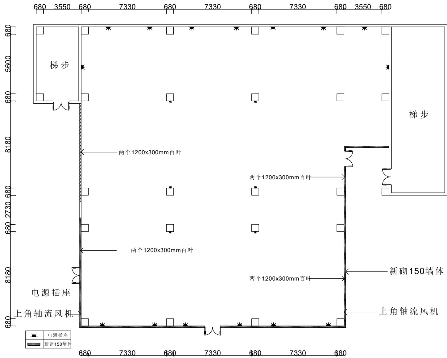
卫健院车间平面布局图
